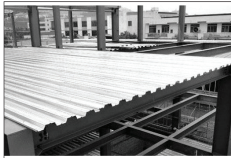
Tablier métallique et toiture métallique.
