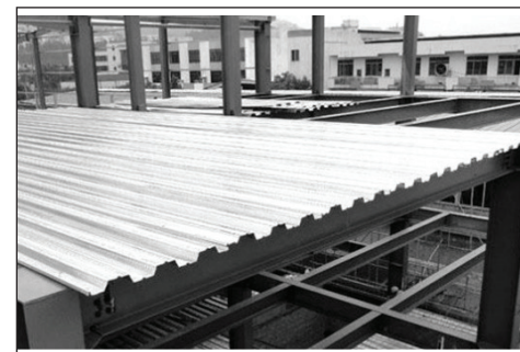
Cubierta de acero y techos de metal
