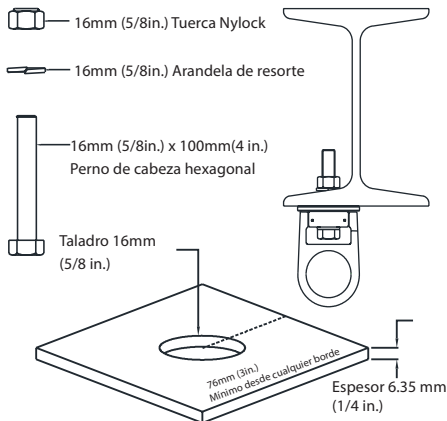
Anclaje basculante de punto único para estructura de Metal (DXFP843102)
